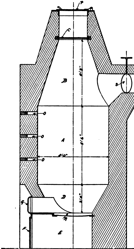
FIG. 11. — BISCHOF PRODUCER.
