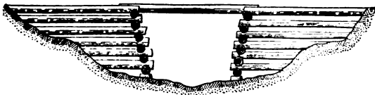
FIG. 56.—Log Bridge.
