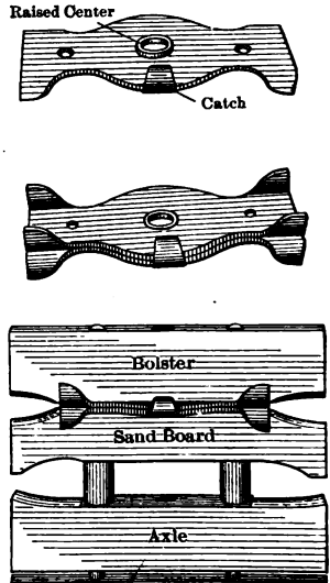
FIG. 144.—Bolster plates.
