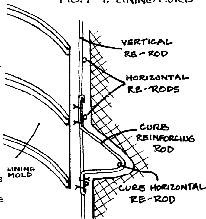
FIG. 7-4. LINING CURB
