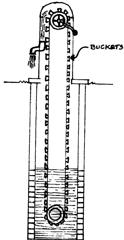
FIG. VII-11. BUCKET PUMP
