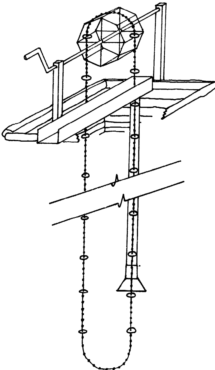
FIG. VII-12. CHAIN PUMP
