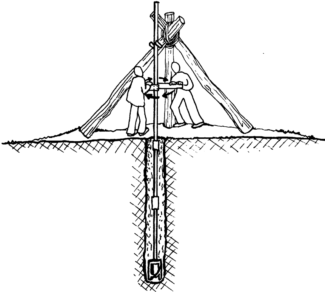
FIG. 12-1. HAND AUGERING
