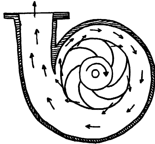
FIG. VII-13. CENTRIFUGAL PUMP
