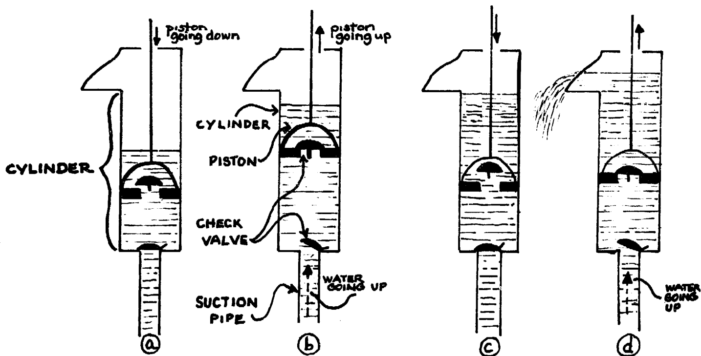
FIG. VII-1. PUMP ACTION
