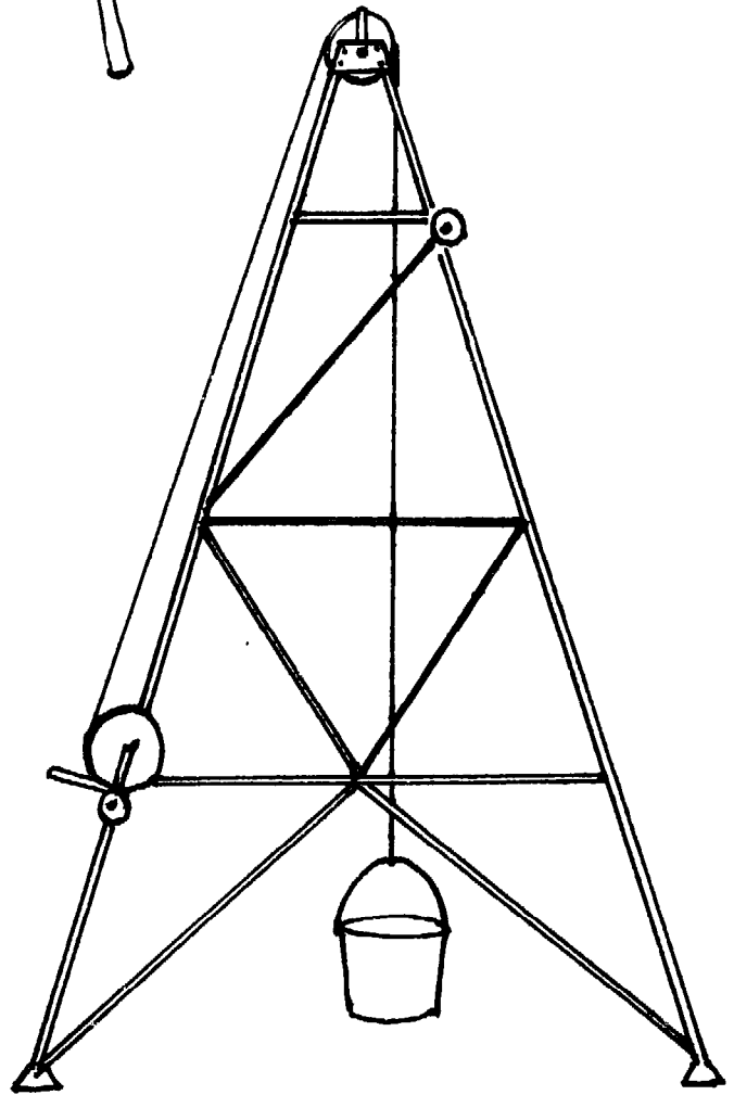
FIG. 5-6. HEADFRAME
